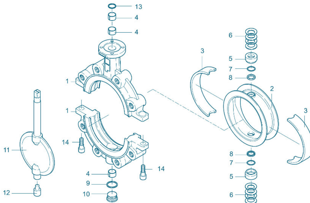
PTFE přírubová klapka DN 80–200
