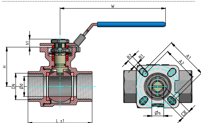
TABULKA ROZMĚRŮ TYP KH 300 / 310-ETE MEASURING GUIDE TYPE KH 300 / 310-ETE
