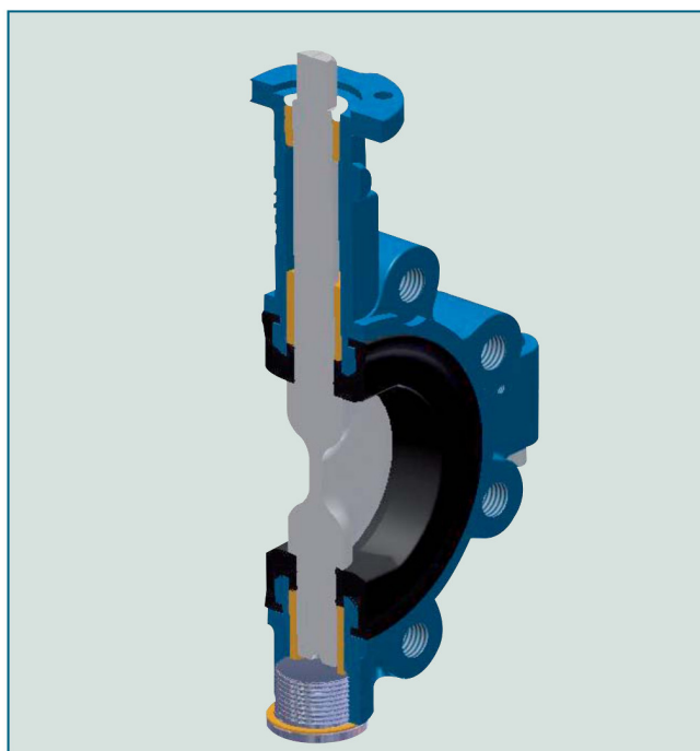
Klapka Z614-A v řezu
